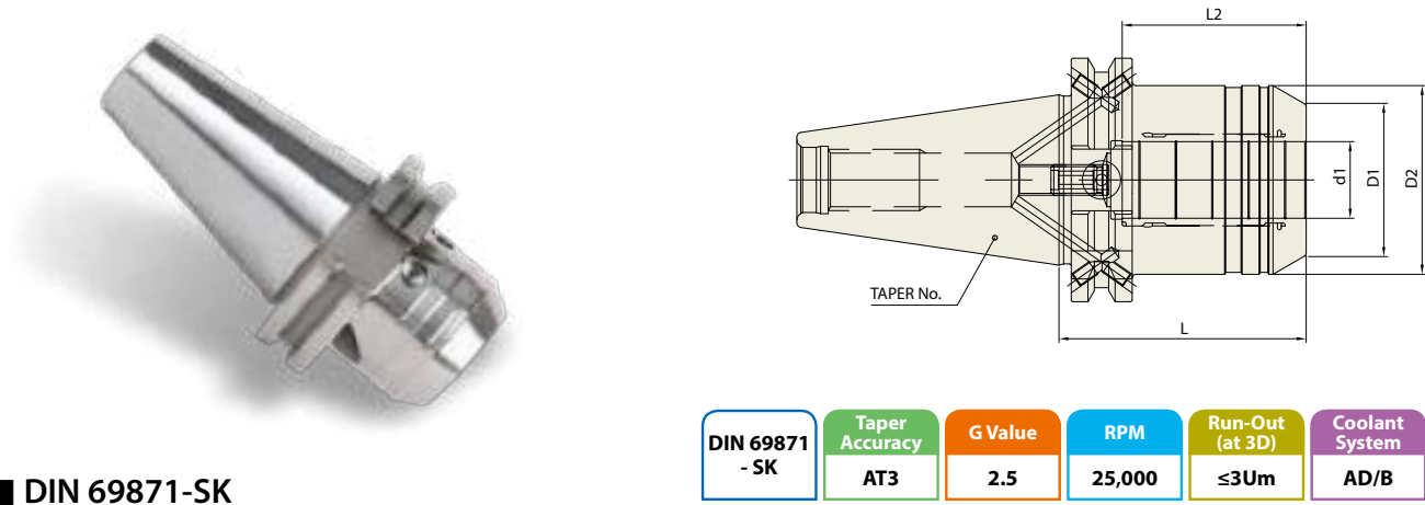
DIN 69871-SK
