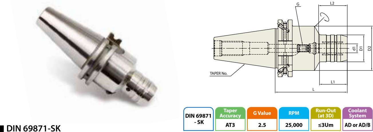
DIN 69871-SK
